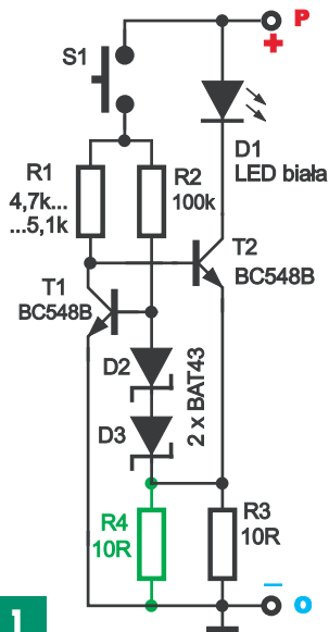
Schemat ideowy
