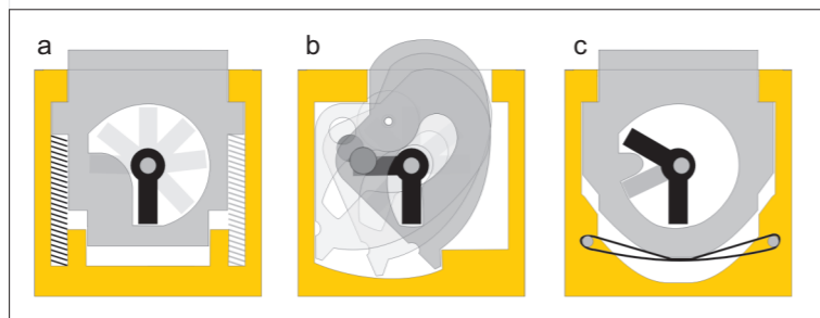
Przykłady zamków do skrzynki pocztowej (3 warstwy sklejk, 40×40 mm) a) ze sprężyną/-nami długopisowymi b) z dwoma magnesami neodymowymi c) z gumkami do warkoczy (małymi)
